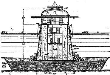
قطاع عرضي
